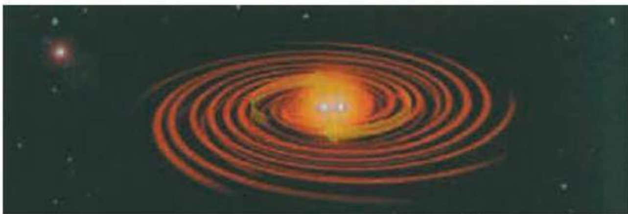
Hai sao neutron đang tiến lại gần nhau theo hình xoáy ốc
